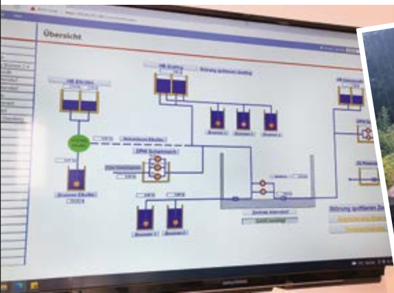
Wasserwerk Übersichtsplan
