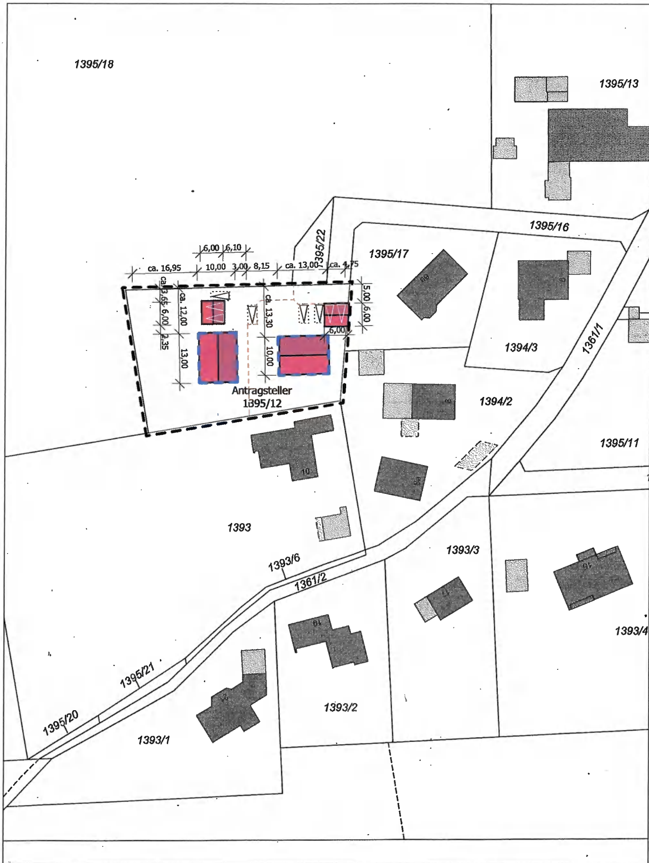
LAGEPLAN M 1/1000
